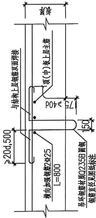
顶板吊环详图
